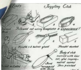
Schéma de fabrication d'une massue Lind, 1920
